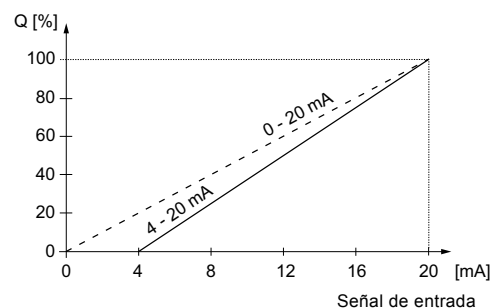
Fig. 10 Control, 0/4 - 20 mA
