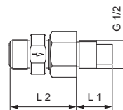
Fig. 38 Unidad de inyección estándar, versión acero inoxidable
