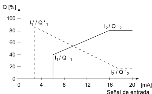
Fig. 11 Escala analógica
