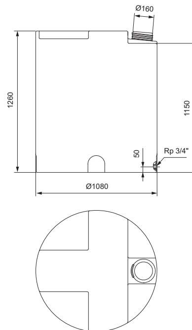
Fig. 57 Tanque cilíndrico, 1000 litros
