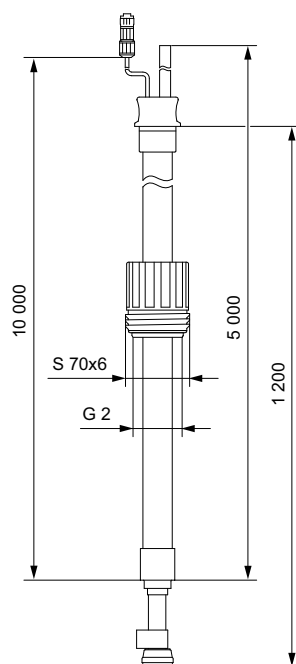
Fig. 36 Línea de aspiración rígida para bidones
