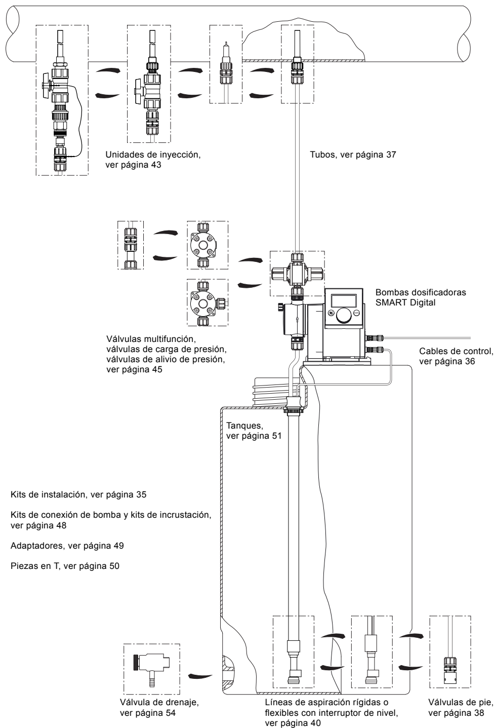
Fig. 23 Bomba SMART Digital con accesorios
