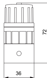
Fig. 28 Válvula de pie, hasta 60 l/h, dimensiones
