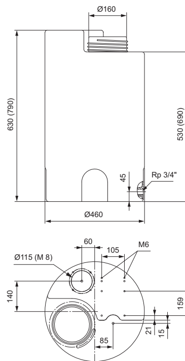
Fig. 53 Tanque cilíndrico, 75 y 100 litros.
