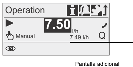
Fig. 16 Pantalla adicional
