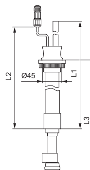
Fig. 34 Línea rígida de aspiración para tanques
