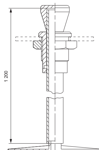
Fig. 60 Mezclador manual, dimensiones
