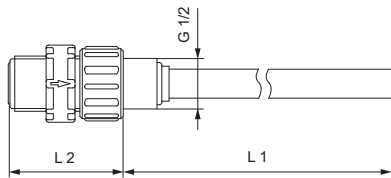
Fig. 37 Unidad de inyección estándar, versión PP, PVC, y PVDF
