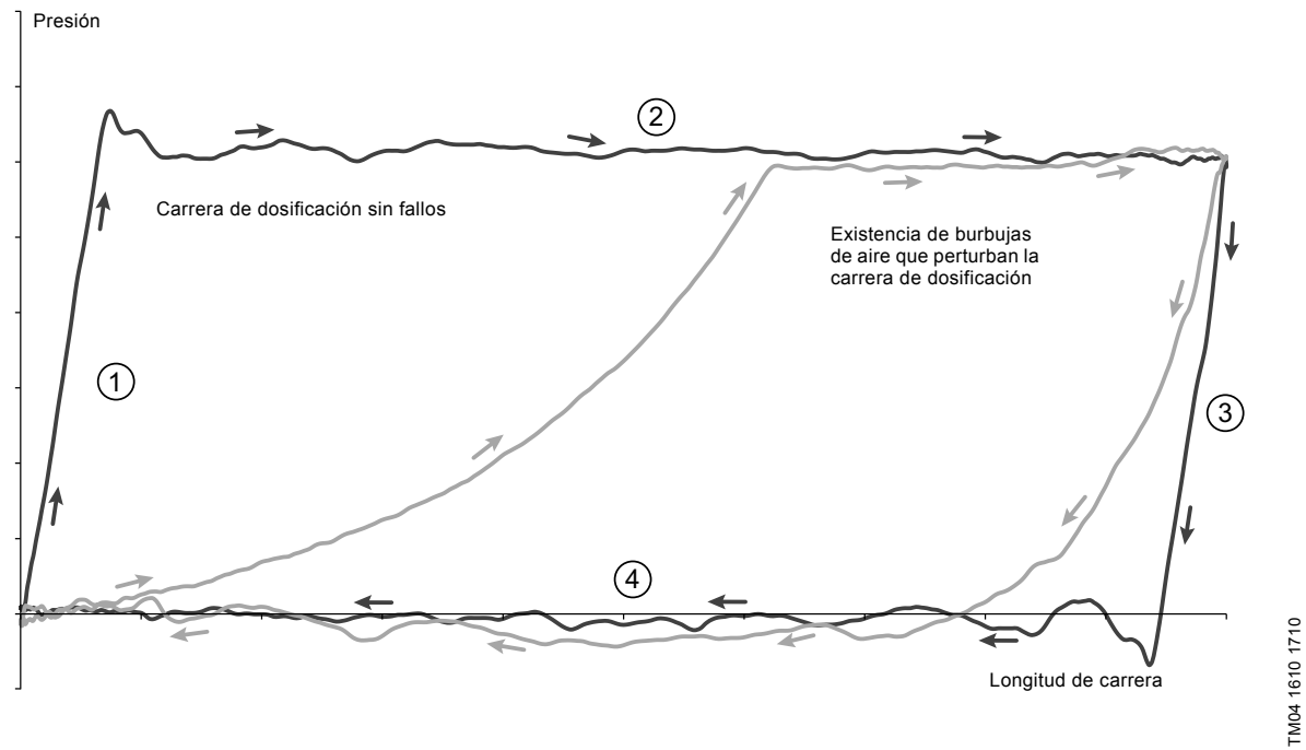
Fig. 18 Gráfico indicador
