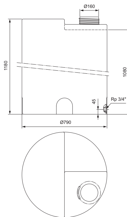
Fig. 56 Tanque cilíndrico, 500 litros
