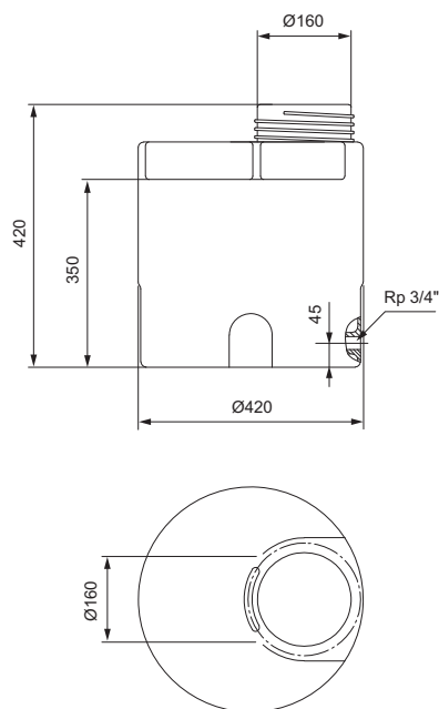
Fig. 52 Tanque cilíndrico, 40 litros
