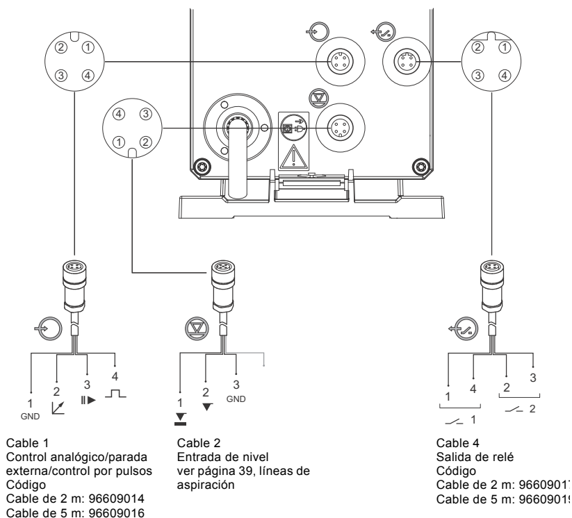
Cable 1: Entrada analógica, parada externa y de pulso
