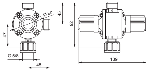
Fig. 44 Válvula multifunción
