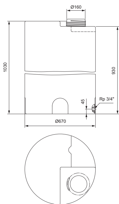
Fig. 55 Tanque cilíndrico, 300 litros
