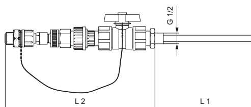
Fig. 41 Unidad de inyección, extraíble para su limpieza
