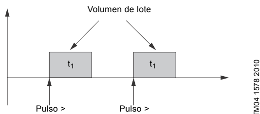
Fig. 12 Control de lote basado en pulso
